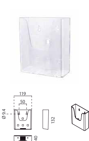
Ref: 13561 Tamaño: A6 10x
